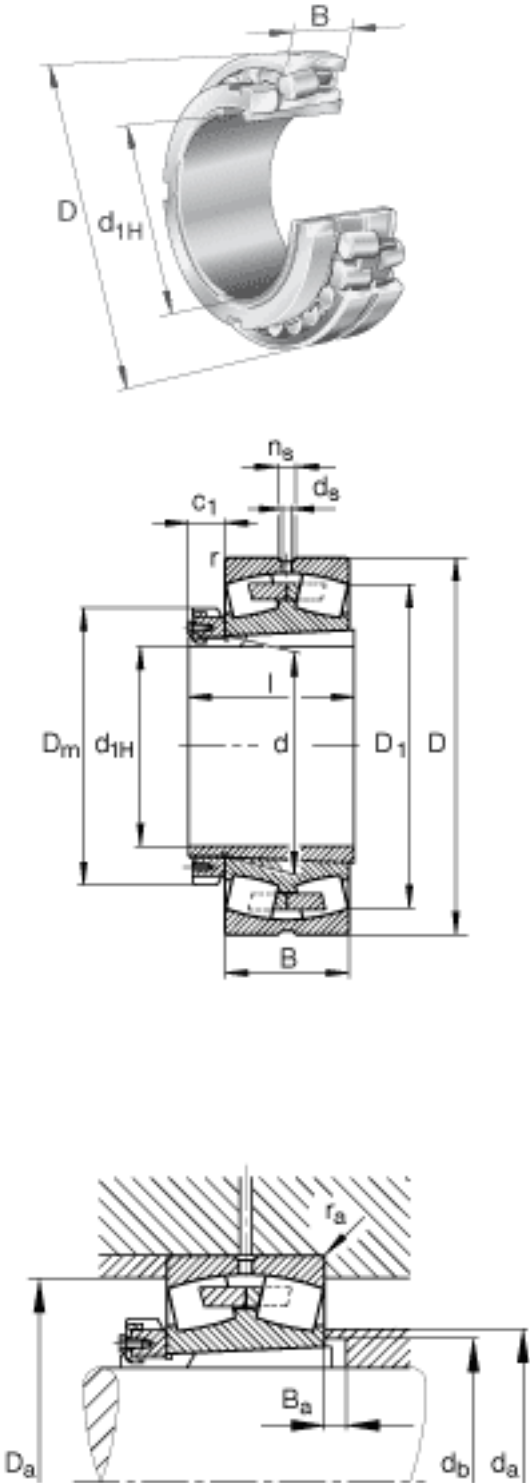
FAG 23168-B-K-MB + H3168图片
