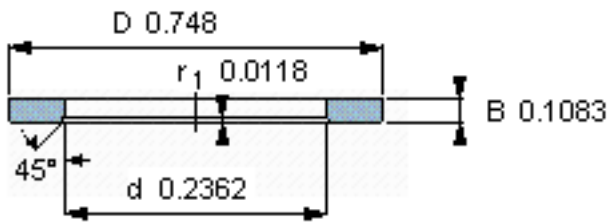
滚道圈
