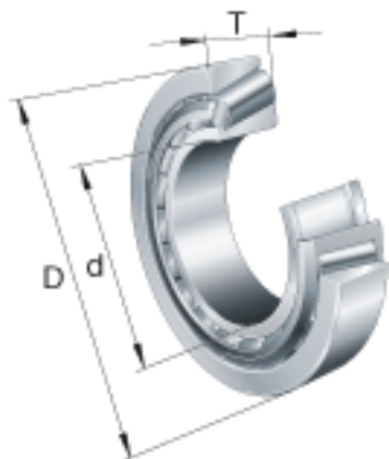
FAG 30310-A图片
