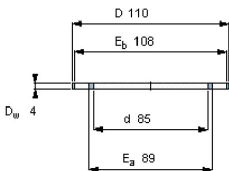
AXK 85110
